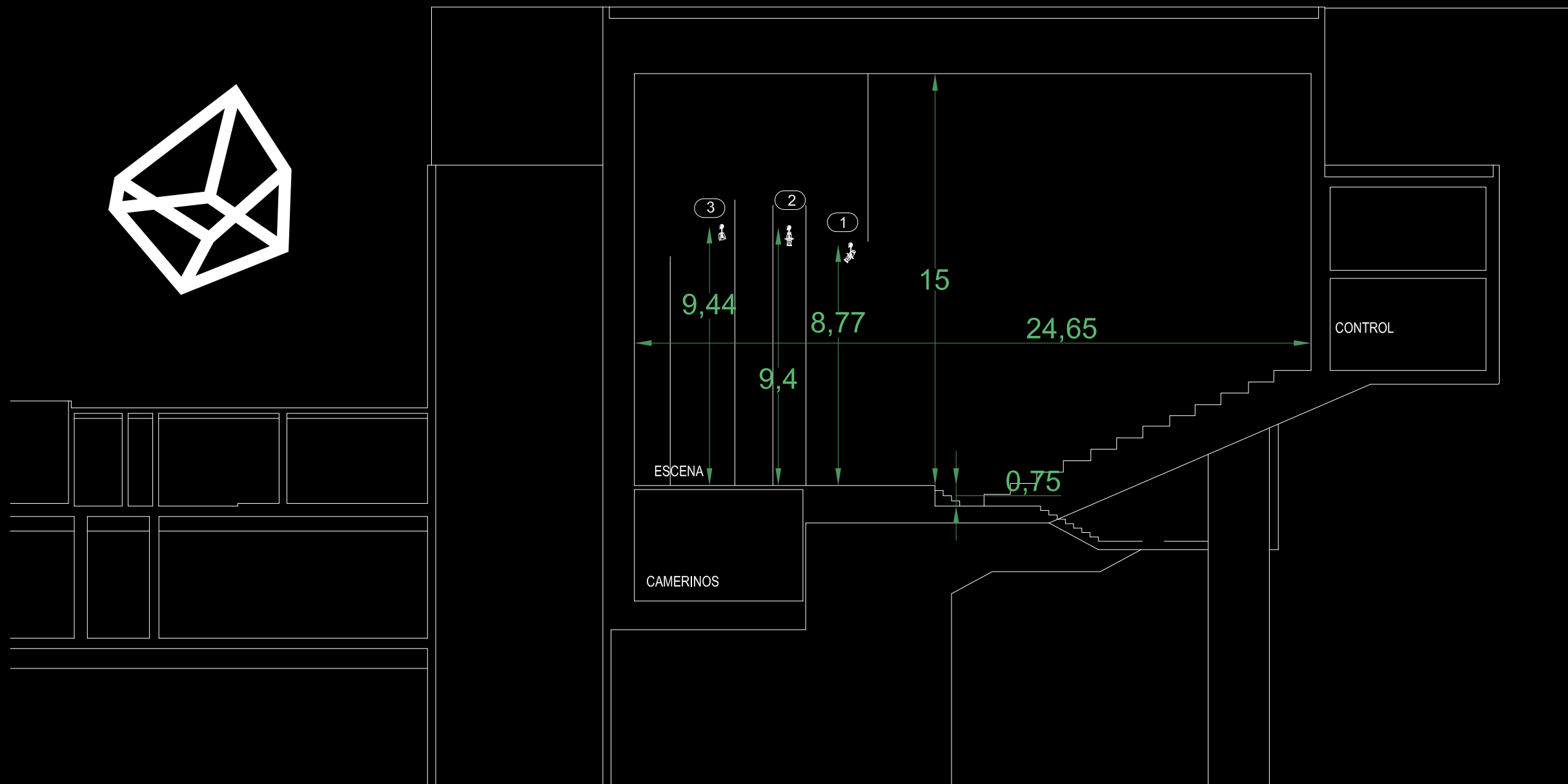
Plano alzado lateral
