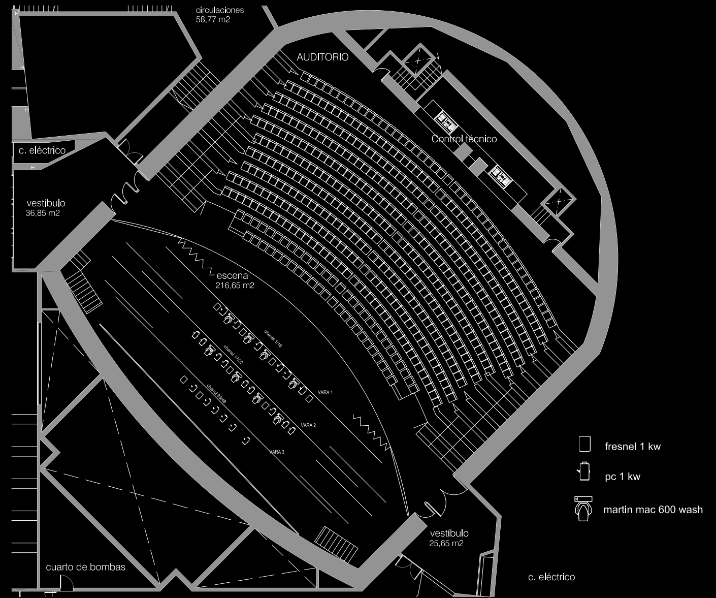
Plano de iluminación
